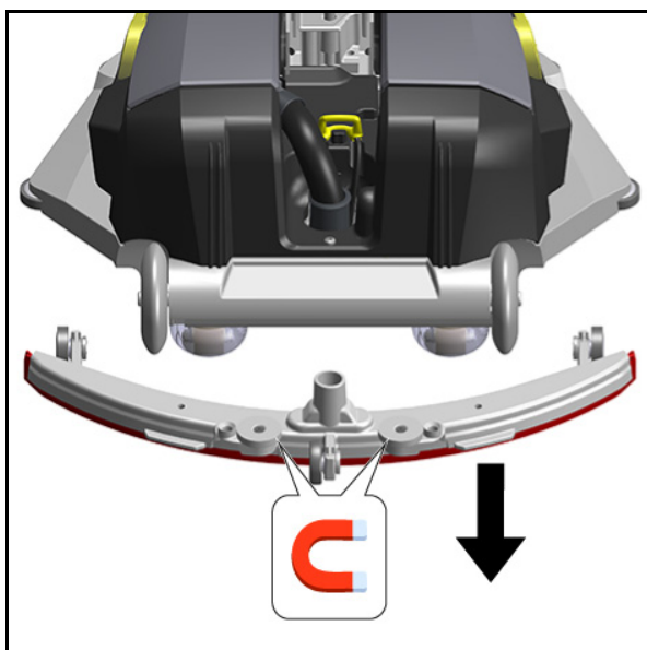
5. ดึงปากดูดออกจากเดือยเพื่อปลดออก
